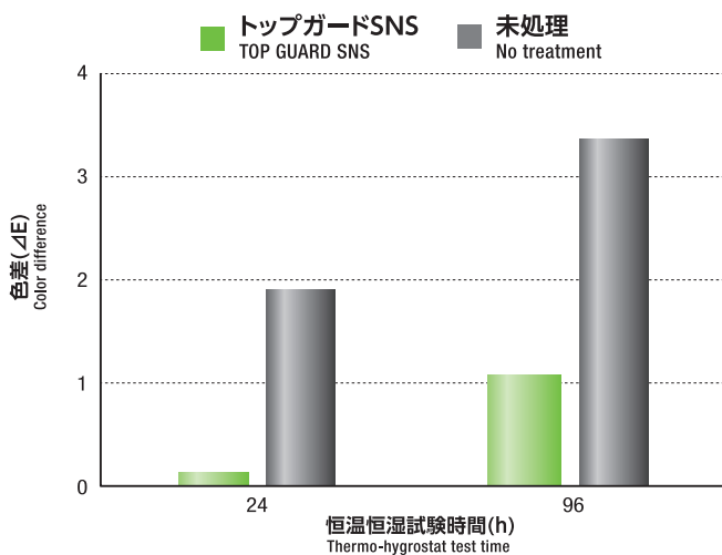
変色度合いの比較 (色差にて評価) Color difference comparison
