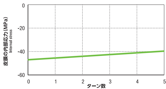
ターン数と皮膜の内部応力の関係 Relationship of metal turn over and internal stress
