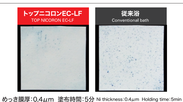
低膜厚でのフェロキシル試験結果 Corrosion comparison by ferroxyl test
