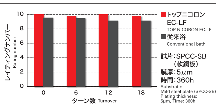
連続使用時の塩水噴霧試験結果 Results of salt spray test by turnover
